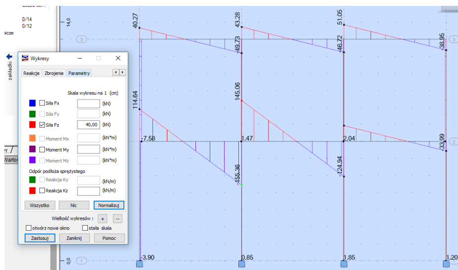
Rys.15. Wykres sił tnących – Fz.
