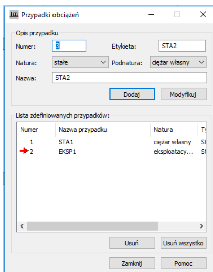
Rys.10. Okno definicji przypadków obciążenia.
