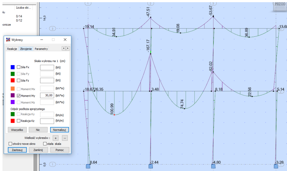
Rys.16. Wykres momentów zginających – My.
