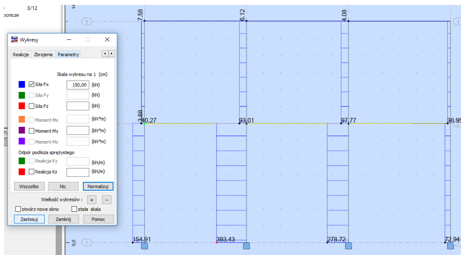
Rys.17. Wykres sił normalnych – Fx.
