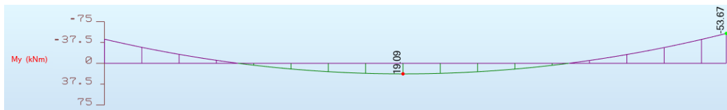
Rys.19. Wykres momentów zginających M_y dla środkowego rygla górnego poziomu – analiza szczegółowa.
