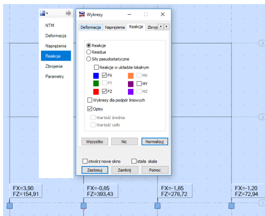
(a) Zaznaczenie reakcji na schemacie ramy.
