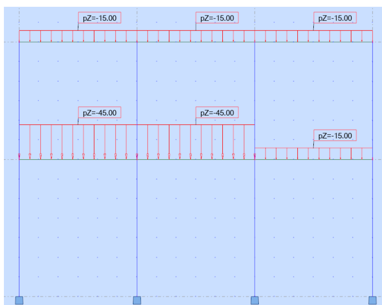
Rys.13. Schemat statyczny ramy w programie ROBOT.
